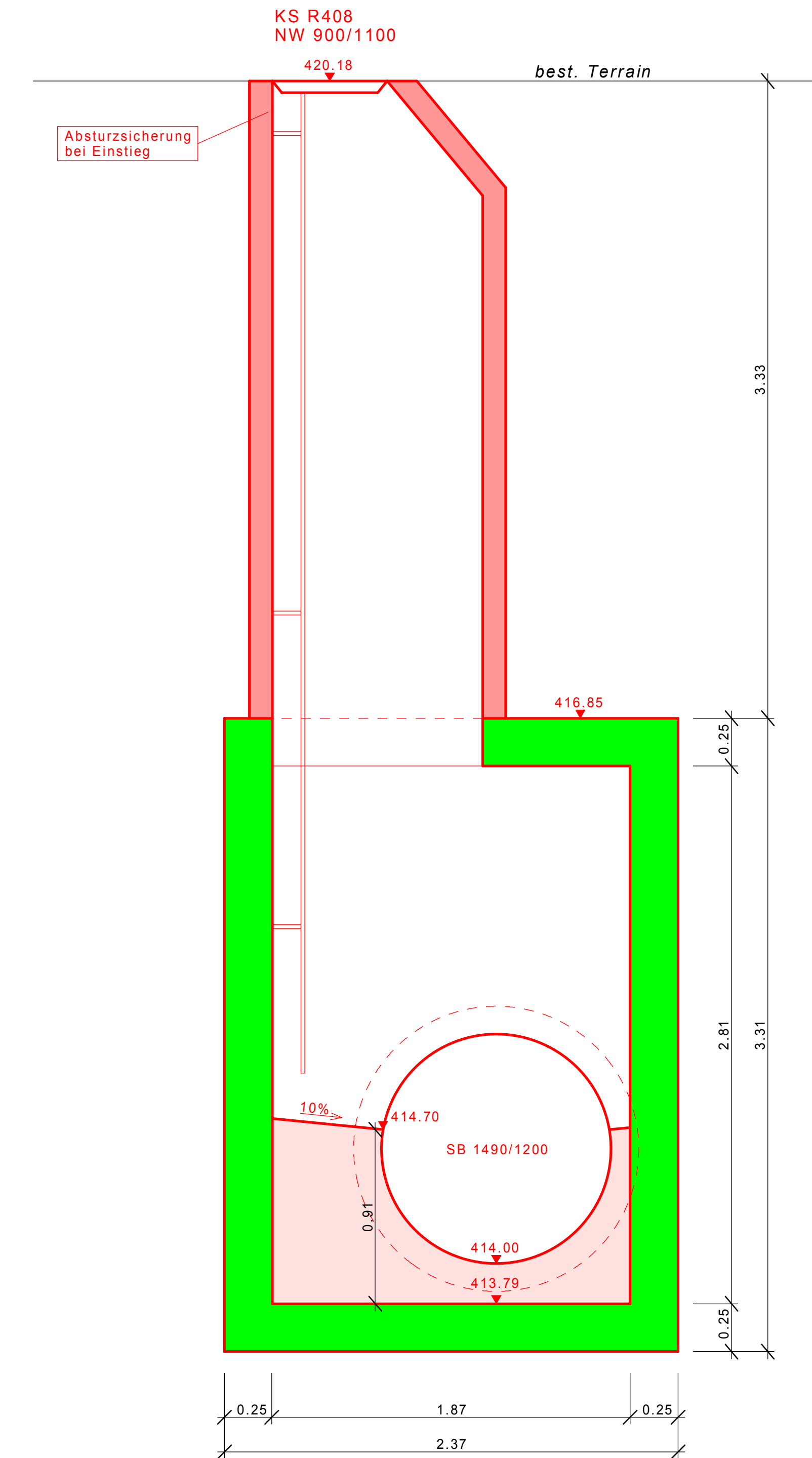
Schnitt A-A 1:20
